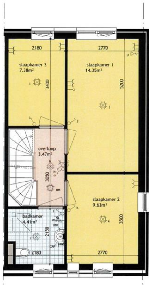
eerste verdieping
